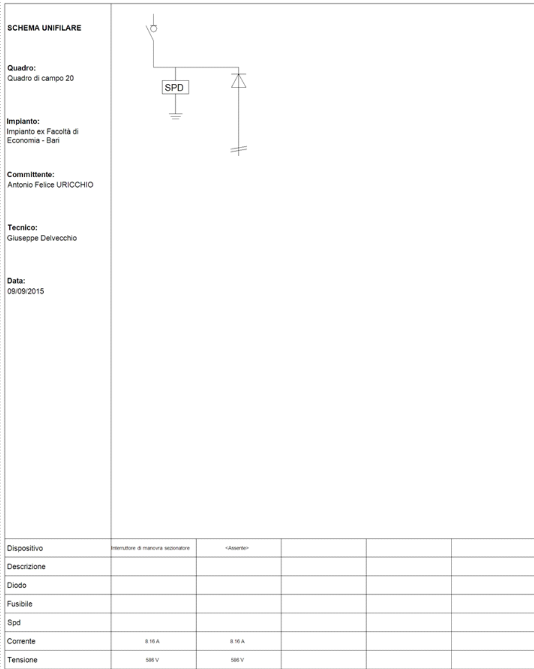
Fig. 27: Schema unifilare quadro "Quadro di campo 20"
