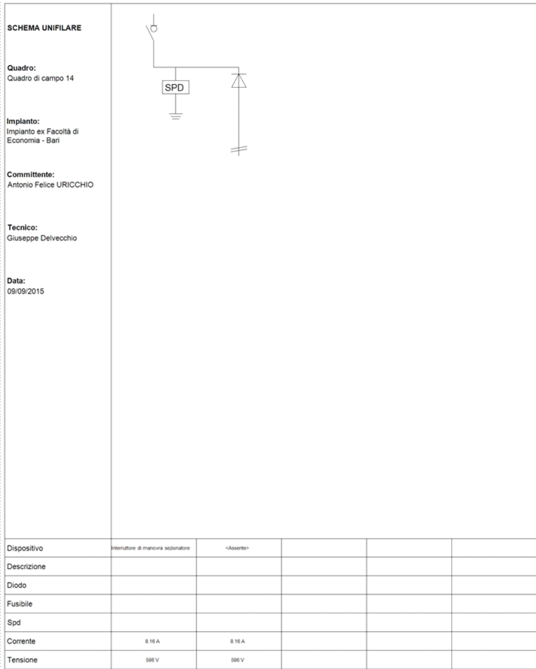
Fig. 21: Schema unifilare quadro "Quadro di campo 14"
