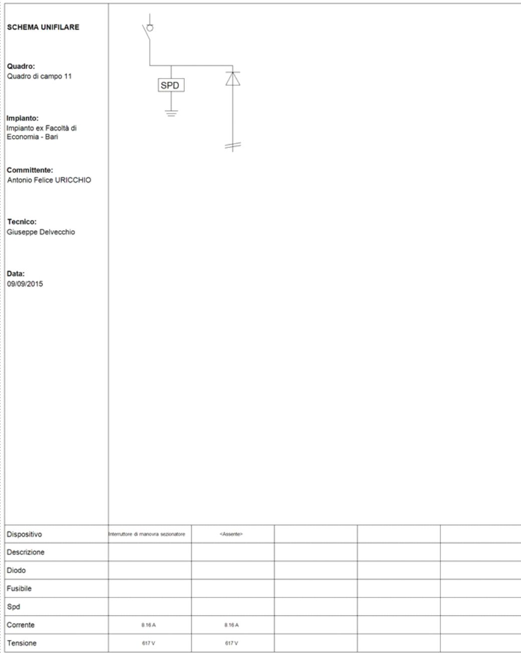
Fig. 18: Schema unifilare quadro "Quadro di campo 11"
