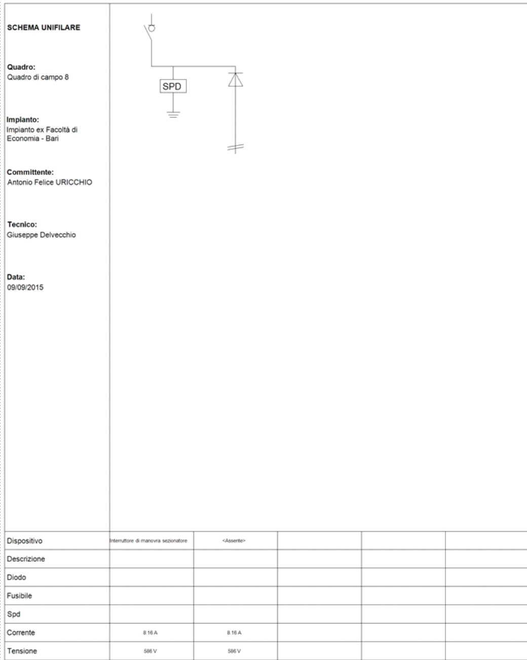
Fig. 15: Schema unifilare quadro "Quadro di campo 8"
