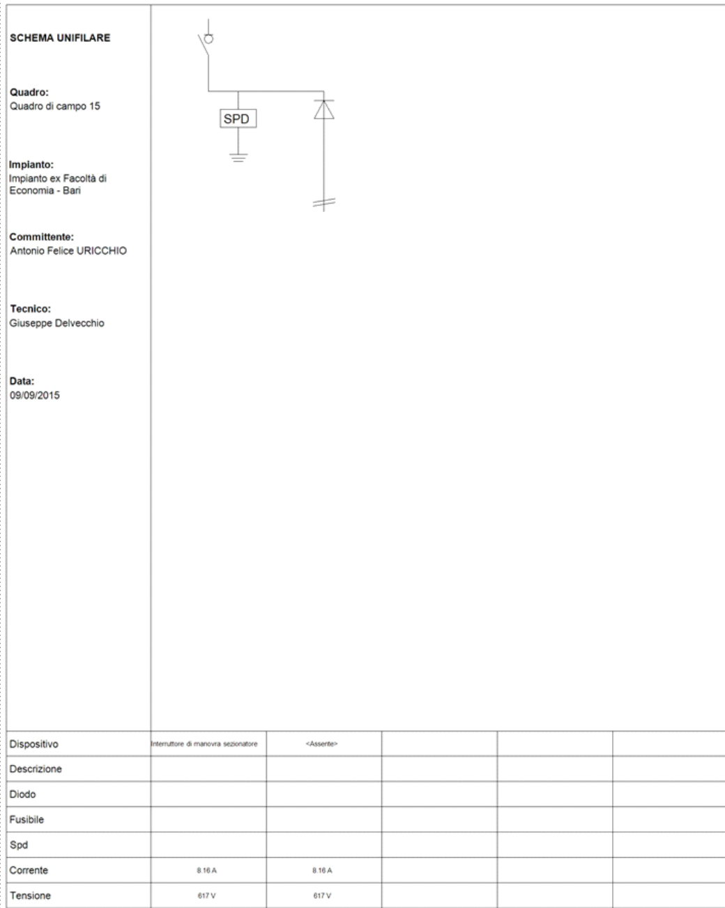
Fig. 22: Schema unifilare quadro "Quadro di campo 15"
