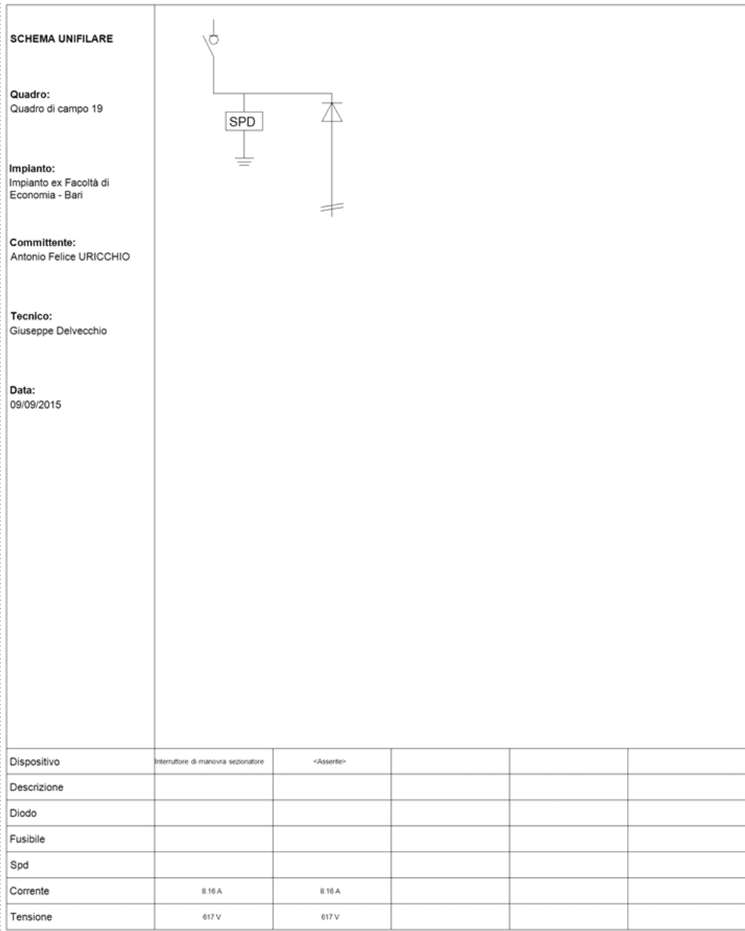
Fig. 26: Schema unifilare quadro "Quadro di campo 19"
