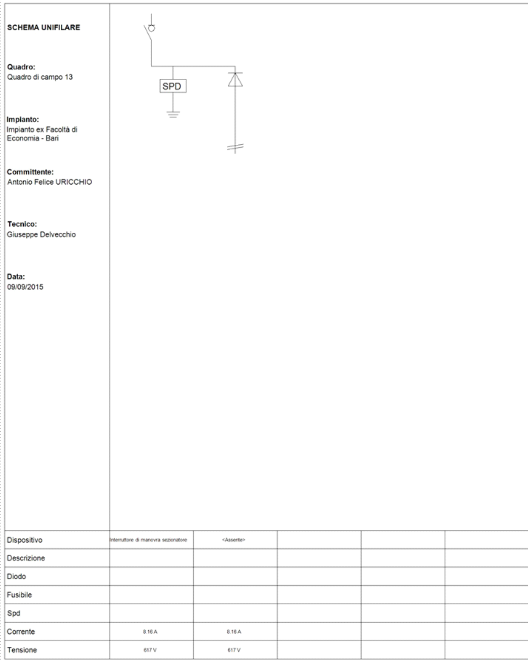
Fig. 20: Schema unifilare quadro "Quadro di campo 13"
